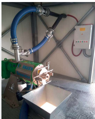
Separátor Bauer
