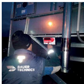
Montáž hladinových čidel, tenzometrů, a uzemnění sil
